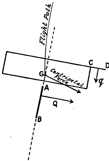
FIG. 78.—Plan.
